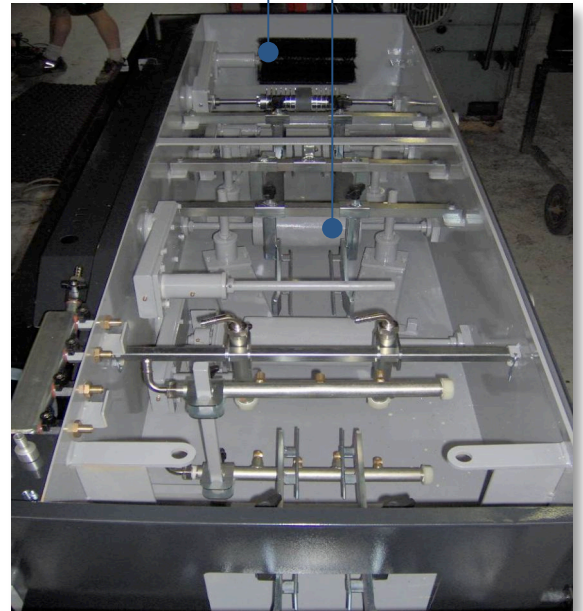
rouleaux entraîneurs
